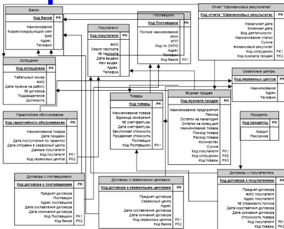
Рисунок 8 – Логическая модель бизнес классов предметной области
